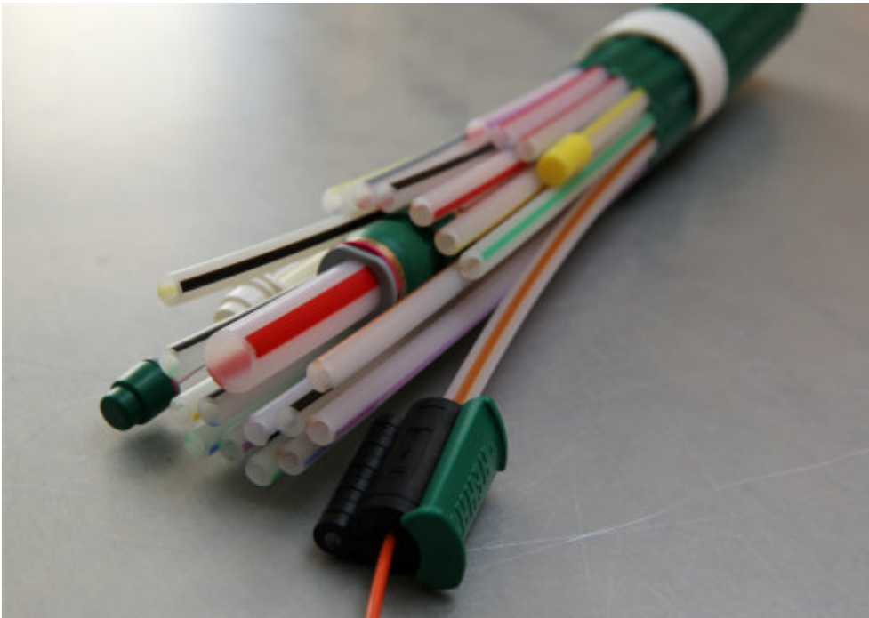
Leerrohrverbund für Glasfaser. (Foto: OBK) Link auf Original-Bild
